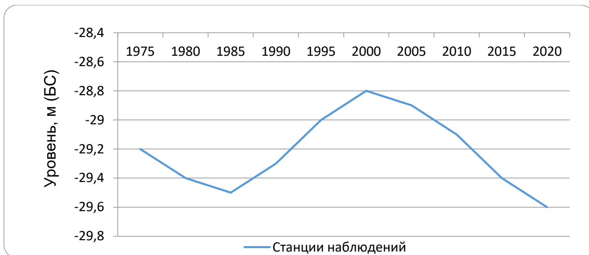
Рисунок 2 - Инструментальные наблюдения
