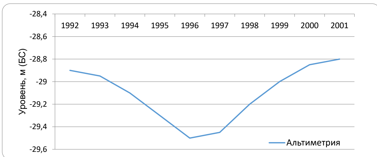
Рисунок 3 - Спутниковая альтиметрия
